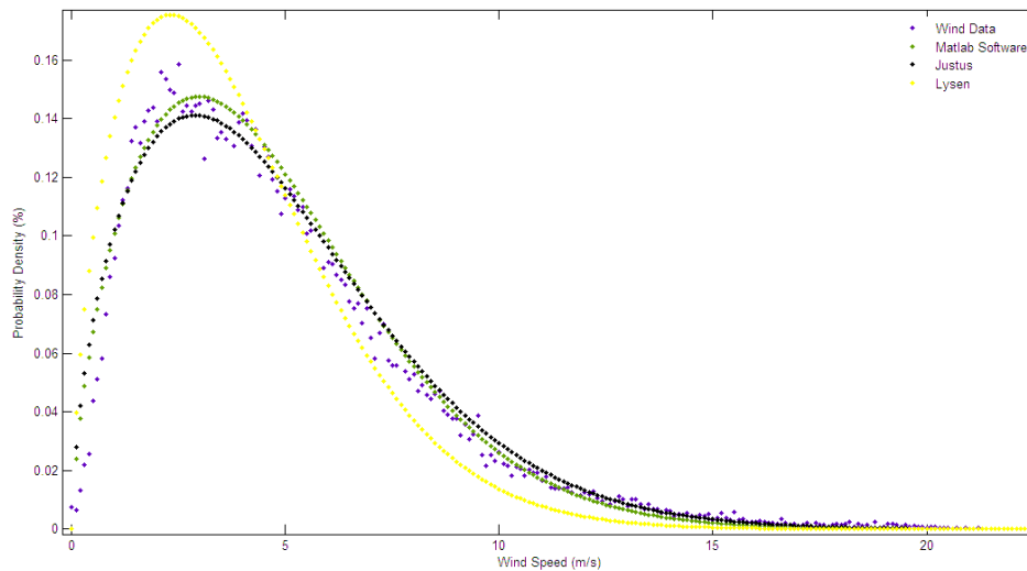
شکل ۵- تابع توزیع ویبول برای ایستگاه سرخس
