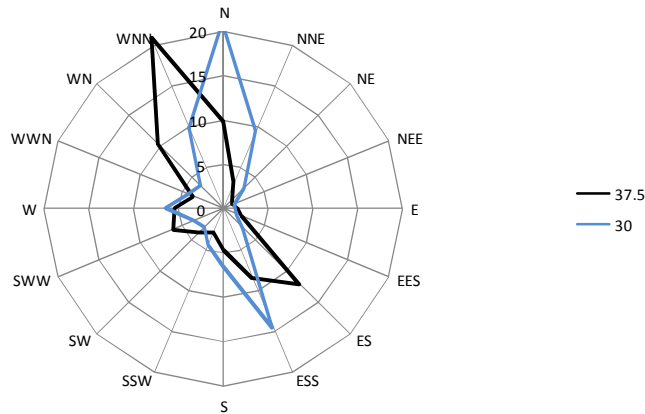
شکل ۴- گلباد سرعت و جهت در ارتفاع ۳۰ متری
